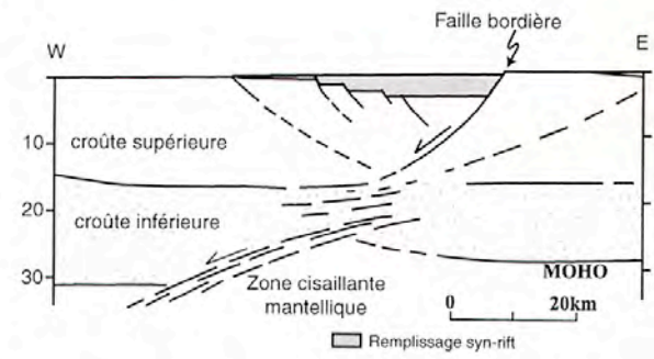
FIG. 10. - Le demi-graben obtenu dans les expériences à une seule DV (sommet) montre des analogies frappantes avec la structure crustale du graben du Rhin telle qu'elle a été déduite des études sismiques [bas : Brun et al. , 1992].
