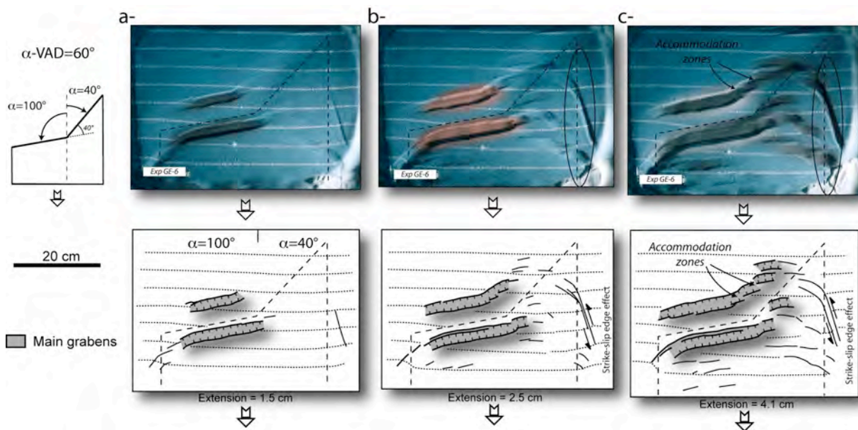
Figure 28: Evolution de la déformation dans le modèle avec \alpha-VAD=60^\circ . Un graben linéaire se développe au niveau du segment sub-orthogonal à l'extension alors que des grabens en échelon se forment le long du segment de VD très oblique à la direction d'extension.
