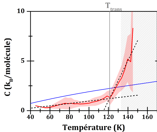
FIGURE 3.12 – Capacité calorifique obtenue pour un agrégat d’eau déprotoné de taille n = 70 , (\text{H}_2\text{O})_{69}\text{OH}^- pour un couple d’énergies dans le référentiel du laboratoire de 38 et 33 eV. La capacité calorifique de la glace macroscopique [98] a été indiquée en bleu. La zone hachurée correspond aux températures supérieures à la température d’évaporation telle que déterminée au paragraphe précédent 3.2.3.
