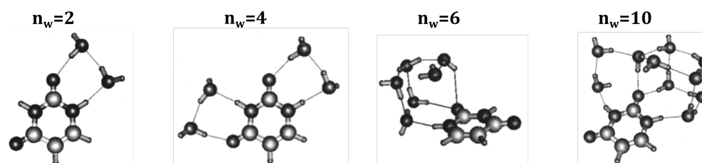
FIGURE 4.12 – Structures calculées par potentiels électrostatiques moléculaires [113]
