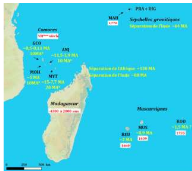
Figure 2. Îles et archipels du Sud-Ouest de l'Océan Indien, avec l'estimation de leur âge géologique (en jaune) et leur date de première colonisation durable (en rouge)
