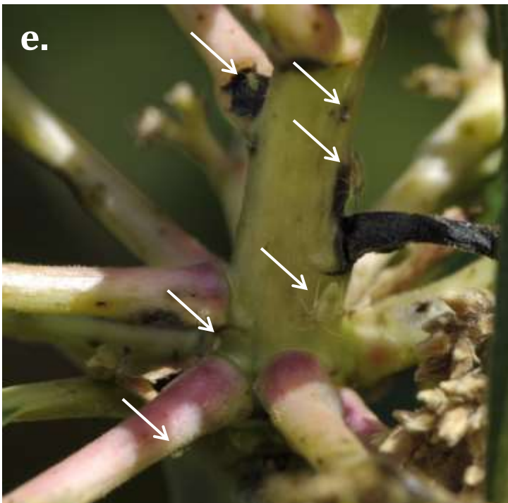
Planche photographique 4. Stades de développement d' Orthops palus (Taylor, 1947) in situ a. 1 er stade larvaire sur un pétiole de manguier ; b. 5 ème stade larvaire sur une tige de manguier ; c. adulte sur un pétiole de manguier ; d. adulte sur une inflorescence de manguier ; e. et f. divers stades de développement présents simultanément. Photographies : Morguen Atiama-CIRAD/Antoine Franck-CIRAD
