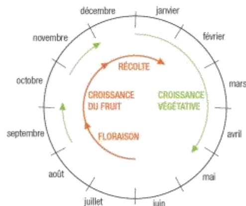
Figure 8. Cycle phénologie du manguier ( Mangifera indica L.) de la variété Cogshall à La Réunion Cycle établi à partir d'observations sur des plants dans la zone Sud de l'île (St-Pierre) (D'après Vincenot et Normand, 2009)
