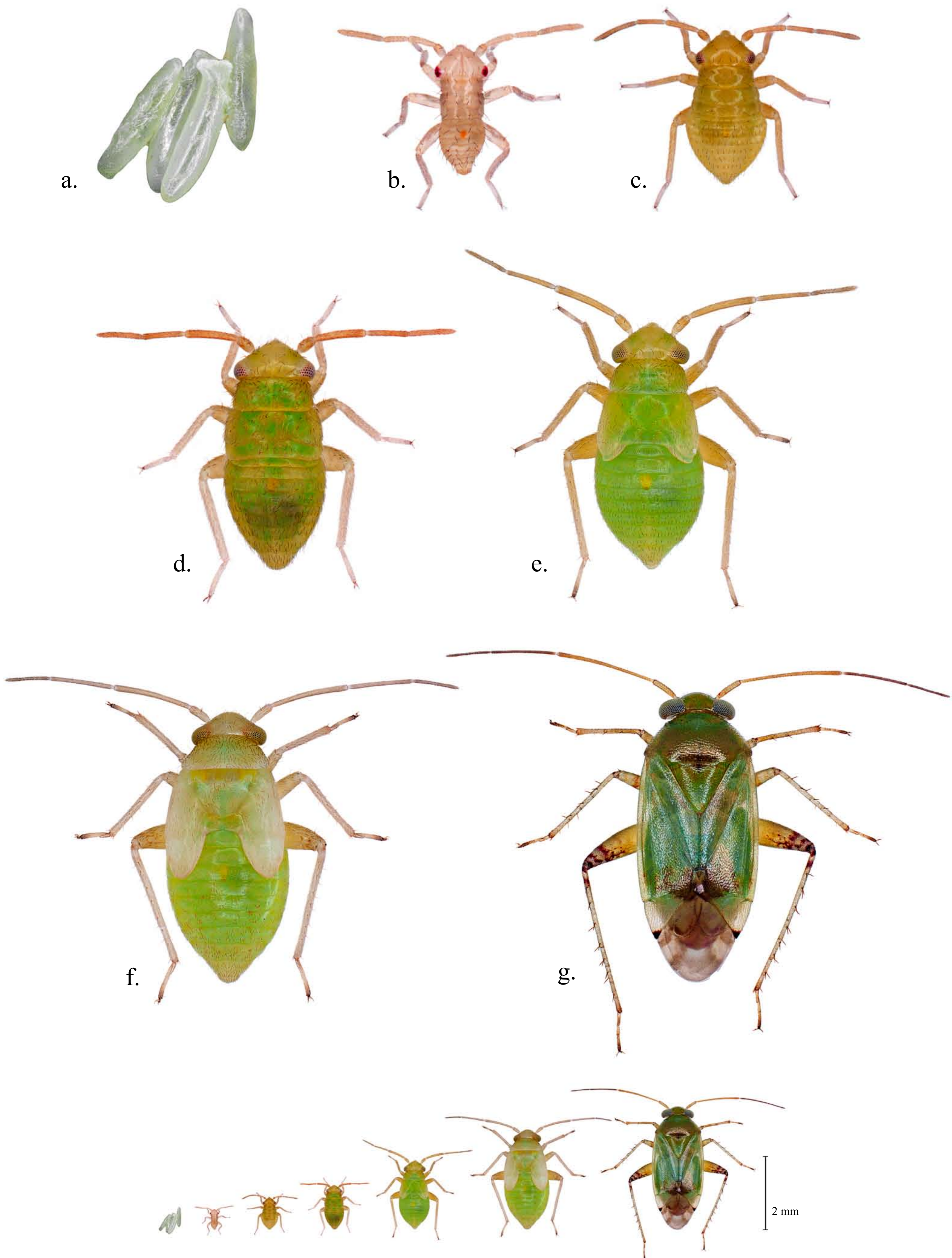
Planche photographique 1. Stades de developpement d' Orthops palus (Taylor, 1947) a. oeufs; b. 1 er stade larvaire; c. 2 ème stade larvaire; d. 3 ème stade larvaire; e. 4 ème stade larvaire; f. 5 ème stade larvaire; g. adulte Photographies : Cédric Ajaguin Soleyen-CIRAD; Infographie : Antoine Franck-CIRAD
