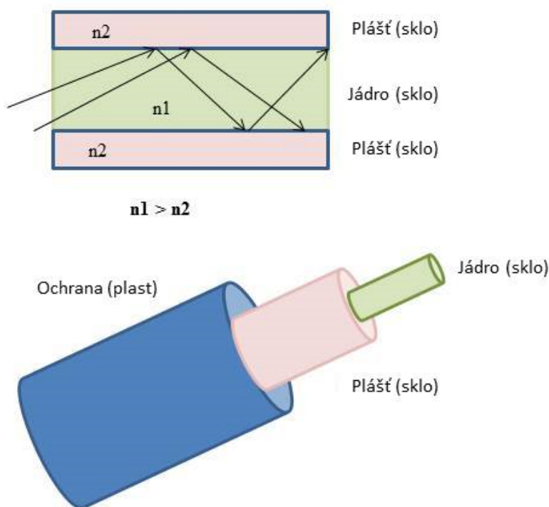
Obr. 13. Optické vlákno.
