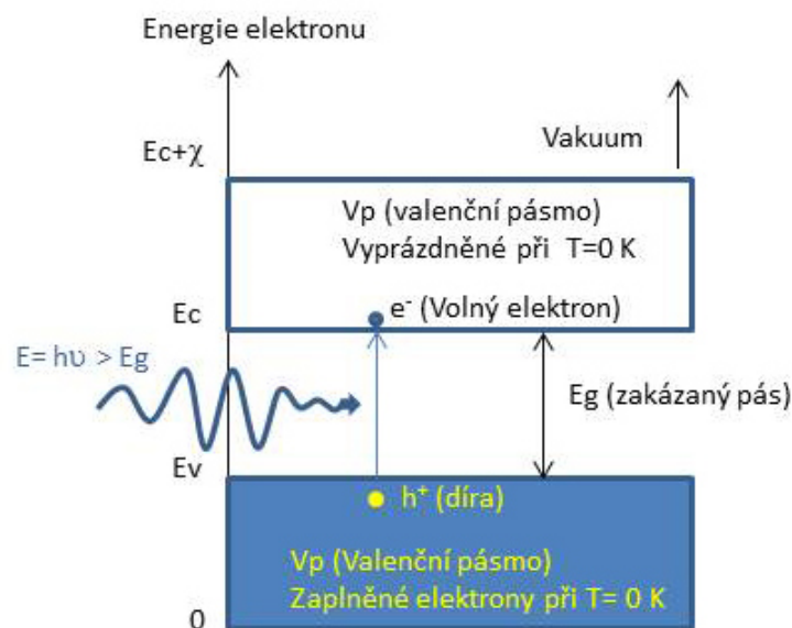
Obr. 6. Pásmový diagram a znázornění mechanismu absorpce fotonu.
