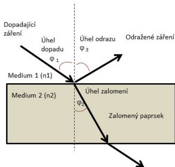
Obr. 2. Úhel zalomení a odrazu paprsku.
