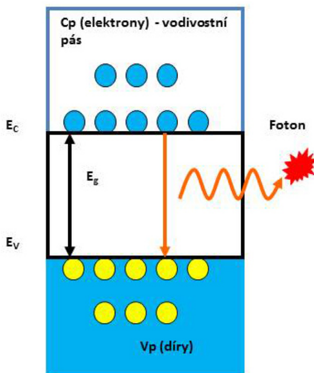
Obr. 7. Emise fotonu.
