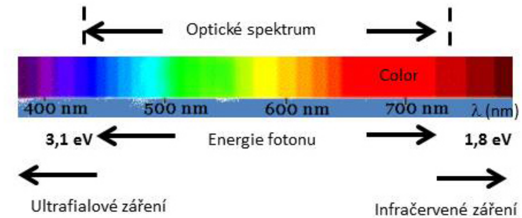
Obr. 1. Optické spektrum.
