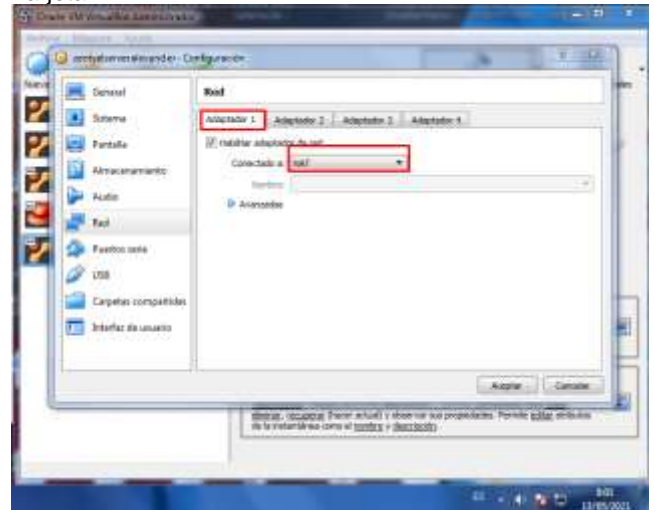
Figura 6: Instalación Zentyal 6.2
