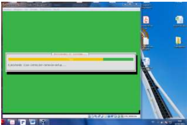
Figura 24: Instalación Zentyal 6.2
