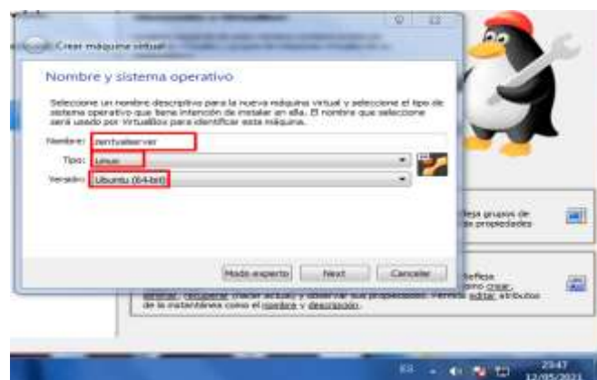
Figura 2: Instalación Zentyal 6.2
