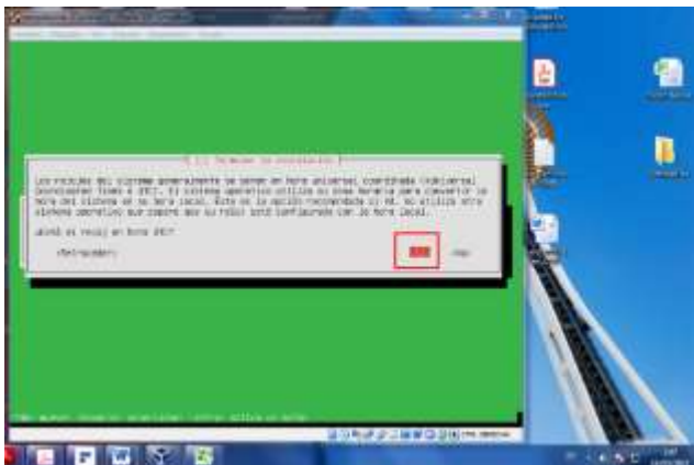
Figura 25: Instalación Zentyal 6.2
