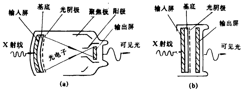
图 1 第一代 X 射线像增强器结构
