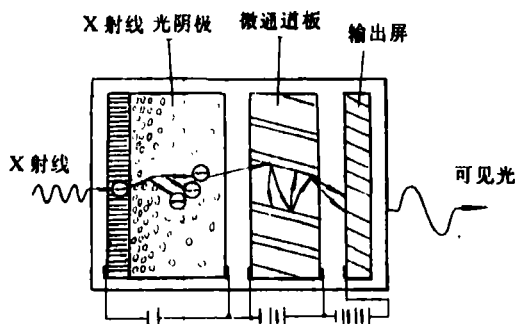
图 5 一次转换器件结构和工作原理
