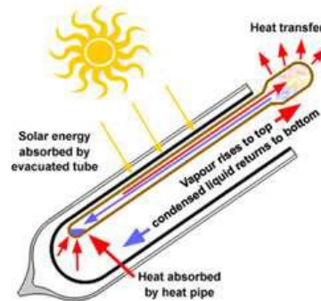
Figura 6. Detalle tubo de calor heat pipe.
