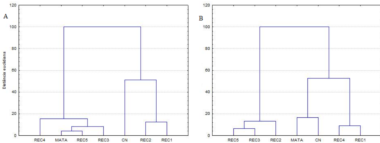
Figura 1- Dendrograma de distância euclidiana com base no DMPs, DMPu e IEA do solo nas áreas em restauração ecológica, vegetação nativa e cultivo de cana-de-açúcar. (A) Camada 0,00-0,10 m, (B) Camada 0,10-0,20 m. REC1 (área em restauração ecológica 1), REC2 (área em restauração ecológica 2), REC3 (área em restauração ecológica 3), REC4 (área em restauração ecológica 4), REC5 (área em restauração ecológica 5), CN (Cana-de-açúcar), MATA (fragmento de vegetação nativa de Floresta Estacional Semidecídua).
