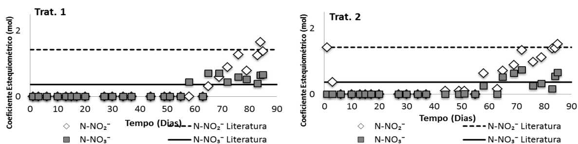
FIGURA 2. Acompanhamento dos coeficientes estequiométricos das formas \text{NO}_2^- e \text{NO}_3^- . Trat.1 (Tratamento com Glicerol), Trat.2 (Tratamento com Leite Desnatado). Linha tracejada: 1,43 mols, valor estequiométrico de \text{NO}_2^- para reação ANAMMOX (SCHIERHOLD NETO et al. , 2006). Linha Contínua: 0,37 mols, valor estequiométrico de \text{NO}_3^- para reação ANAMMOX (SCHIERHOLD NETO et al. , 2006).
