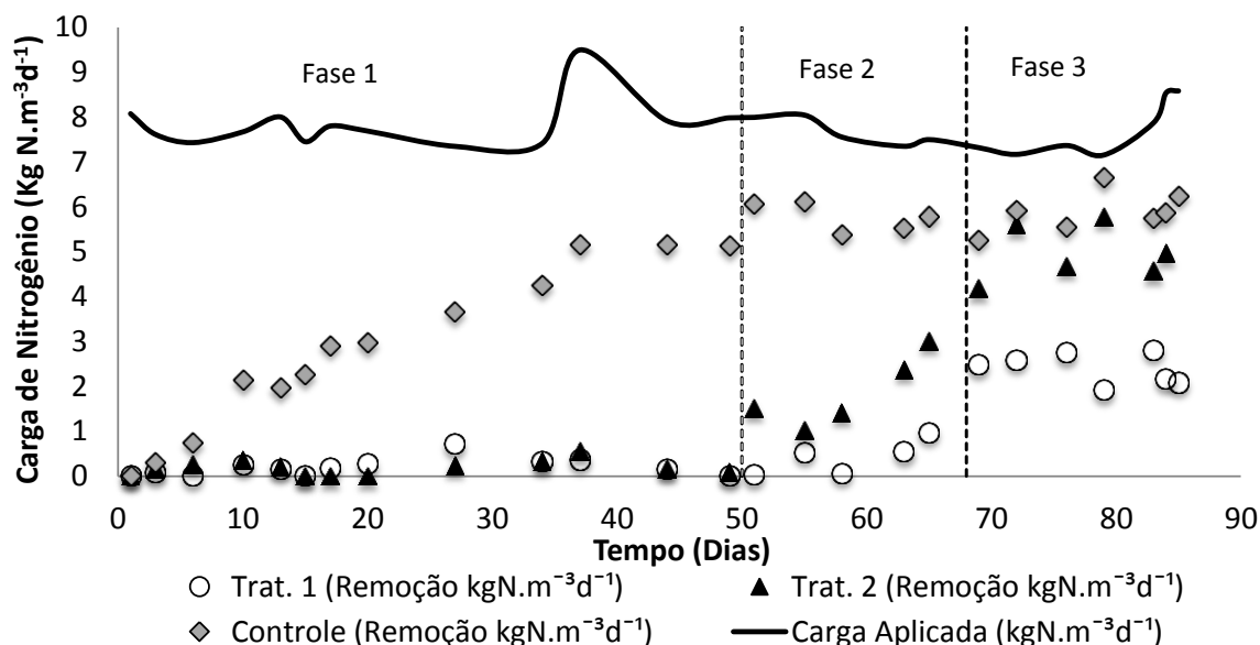
FIGURA 1. Acompanhamento das cargas de nitrogênio aplicadas e removidas. Trat.1 (Tratamento com Glicerol), Trat.2 (Tratamento com Leite Desnatado).
