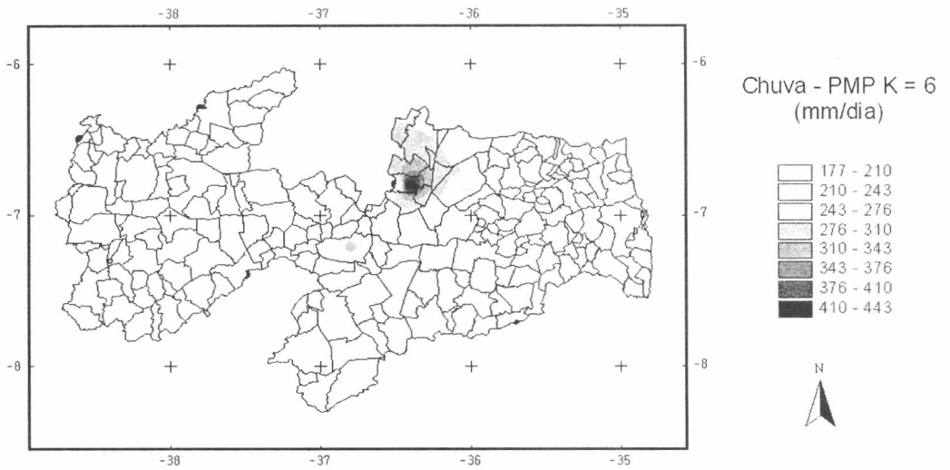
FIGURA 6. ISOLINHAS DE PRECIPITAÇÃO MÁXIMA POSSÍVEL (PMP) COM UM PERÍODO DE RETORNO DE 1000 ANOS (K=6) ESTIMADA USANDO A TÉCNICA DE HERSHFIELD, PARA O ESTADO DA PARAÍBA
