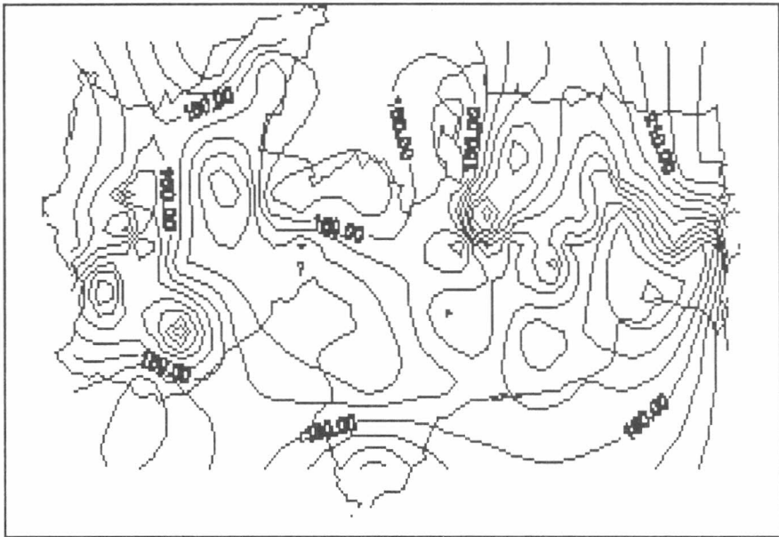
FIGURA 3. REPRESENTAÇÃO ESPACIAL DAS PRECIPITAÇÕES MÁXIMAS DIÁRIAS ANUAIS OBSERVADAS (PMDAO)
