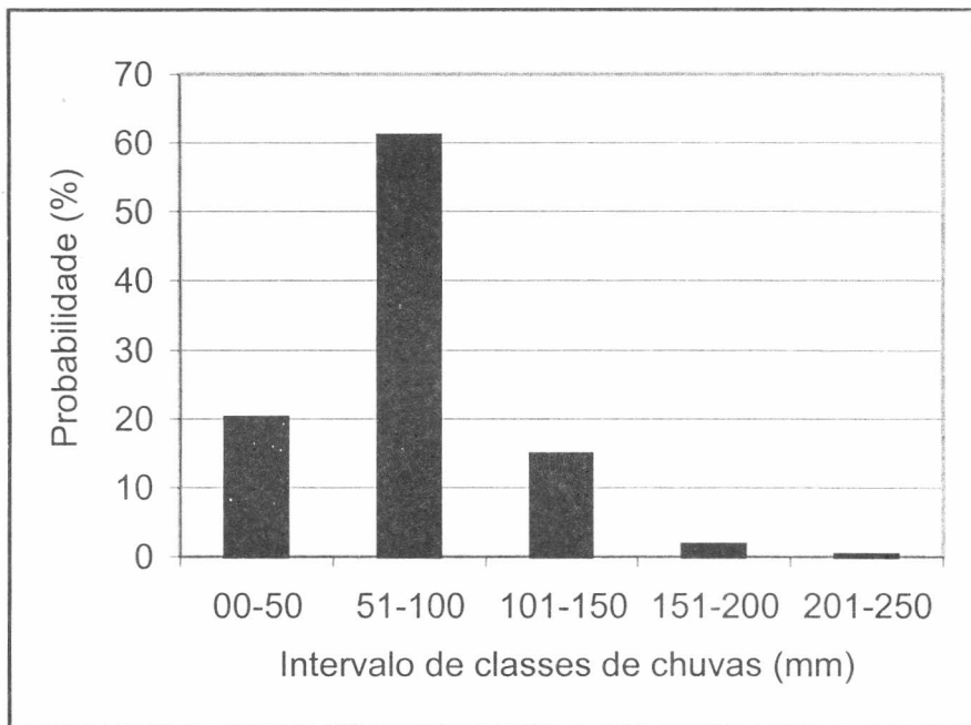
FIGURA 2. HISTOGRAMA DE FREQUÊNCIA DAS PRECIPITAÇÕES MÁXIMAS DIÁRIAS ANUAIS (PMDA), PARA O ESTADO DA PARAÍBA.
