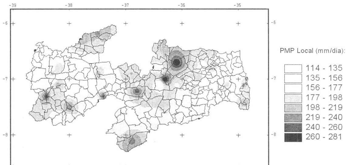
FIGURA 5. ISOLINHAS DE PRECIPITAÇÃO MÁXIMA POSSÍVEL (PMP) LOCAL ESTIMADA UTILIZANDO A TÉCNICA DE HERSHFIELD, PARA O ESTADO DA PARAÍBA.
