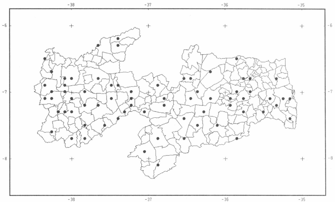
FIGURA 1 - DISTRIBUIÇÃO ESPACIAL DOS POSTOS PLUVIOMÉTRICOS EM ESTUDO
