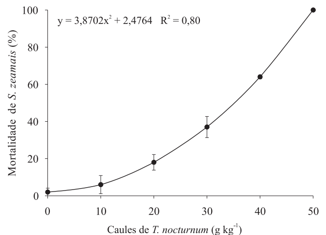
Figura 2. Curva de resposta da mortalidade de adultos de Sitophilus zeamais em razão de concentrações crescentes de segmentos de caules de Tanaecium nocturnum na massa de grãos de milho utilizados na fumigação do milho armazenado.
