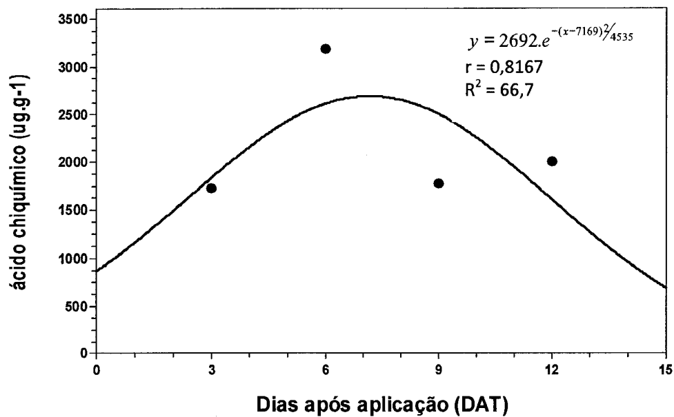
Figura 2: Curva de resposta da concentração de ácido chiquímico em B. plantaginea tratada com Roundup Original a 0,1 L.ha -1 .
