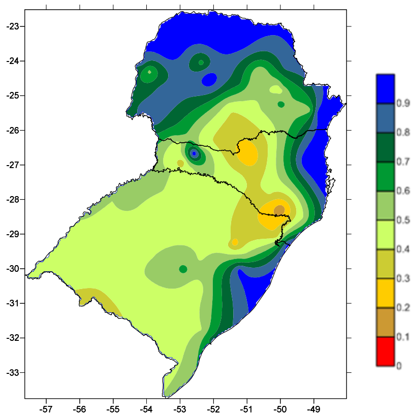
Figura 1. Indicador de sustentabilidade para o trigo na região Sul do Brasil, baseado no risco de geada na floração do trigo, variando de 0 (menor sustentabilidade) a 1 (maior sustentabilidade). Passo Fundo – RS, 2013.
