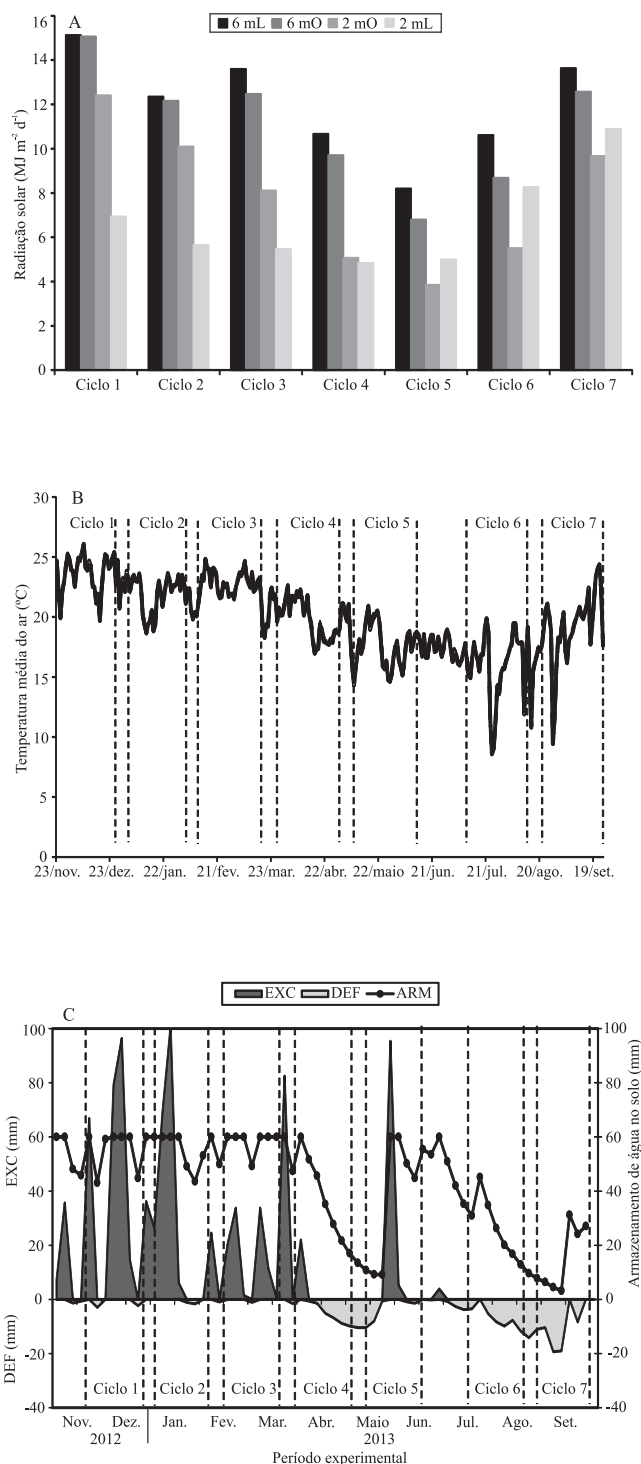
Figura 2. Dinâmica dos fatores ambientais durante o período experimental, nas posições a 6 m do renque leste (6 mL), a 6 m do renque oeste (6 mO), a 2 m do renque oeste (2 mO) e a 2 m do renque leste (2 mL), em sistema silvipastoril. A, radiação solar média; B, temperatura média do ar; C, armazenamento de água no solo (ARM); DEF, deficiência hídrica; e EXC, excedente hídrico.
