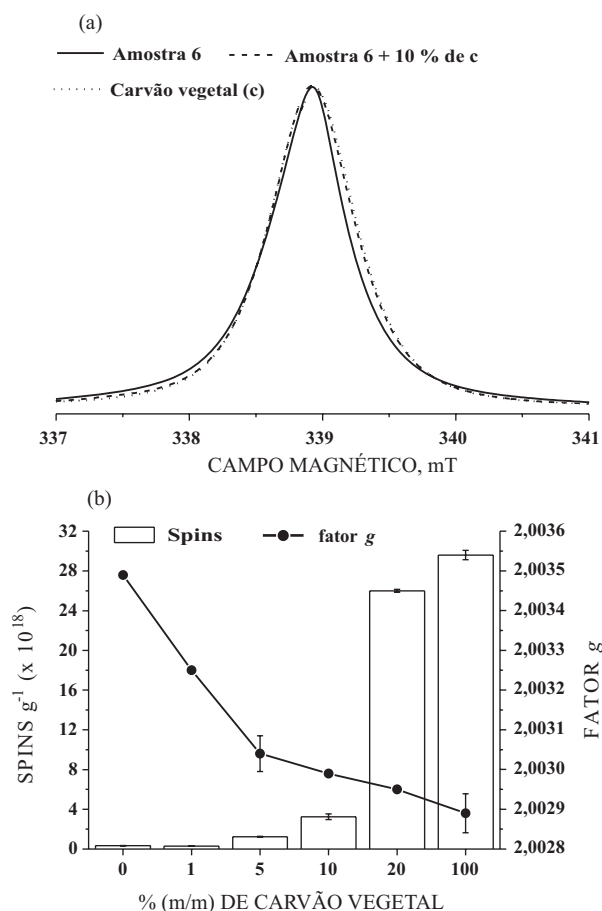
Figura 6. Linhas de absorção normalizadas da amostra 6, da amostra 6 + 10 % (m/m) de carvão vegetal e somente do carvão vegetal (a). Concentração de RLO (em spins g^{-1} de amostra) da amostra 6 e variação do fator g da amostra 7 de acordo com a porcentagem de carvão vegetal adicionado (b).
