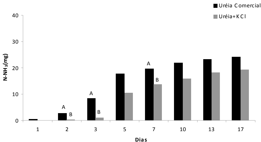
Figura 2 . Perdas acumuladas de amônia (N-NH 3 ) por volatilização em um período de dezessete dias em função da adubação nitrogenada com uréia comercial e fertilizante granulado (mistura de uréia comercial + KCl) sem calagem. Médias seguidas por letras apresentam diferenças significativas, as colunas que não constam letras indicam que as comparações não foram significativas pelo teste de Tukey ao nível de 5%.
