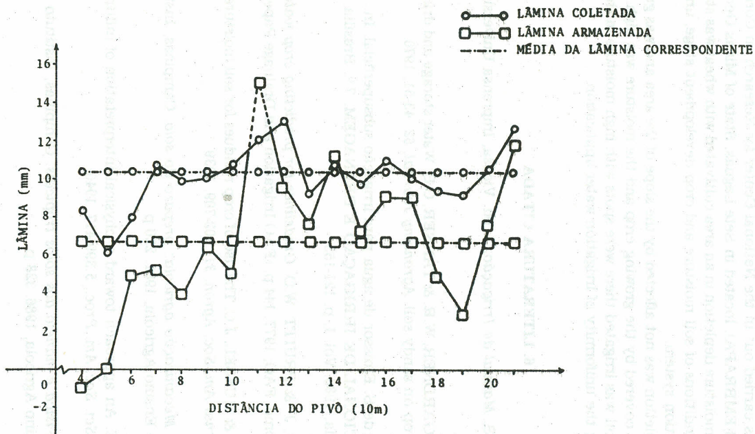
FIGURA 10 - Lâmina coletada e lâmina armazenada na camada de 0 a 60 cm, para o raio um, entre os dias 27 e 28/08, no terceiro estágio de desenvolvimento da cultura (M.S. = 27,1%). Umidade inicial do solo = 36,52% (% em volume).
