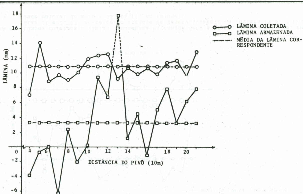
FIGURA 9 - Lâmina coletada e lâmina armazenada na camada de 0 a 60 cm, para o raio um, entre os dias 11 e 12/08, no terceiro estágio de desenvolvimento da cultura (M.S. = 18,2%). Umidade inicial do solo = 35,13% (% em volume).
