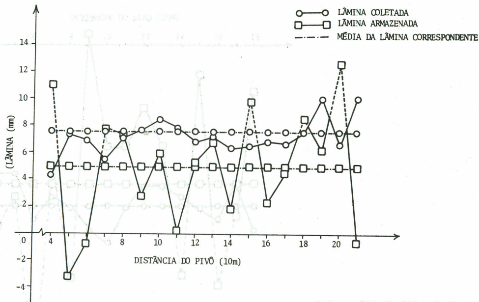
FIGURA 6 - Lâmina coletada e lâmina armazenada na camada de 0 a 60 cm, para o raio quatro, entre os dias 27 e 28/08, no terceiro estágio de desenvolvimento da cultura (M.S. = 27,1%). Umidade inicial do solo = 36,18% (% em volume).
