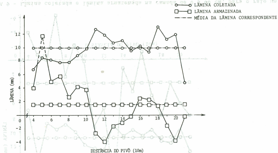
FIGURA 8 - Lâmina coletada e lâmina armazenada na camada de 0 a 60 cm, para o raio um, entre os dias 21 e 22/07, no terceiro estágio de desenvolvimento da cultura (M.S. = 15,2%). Umidade inicial do solo = 35,90% (% em volume).
