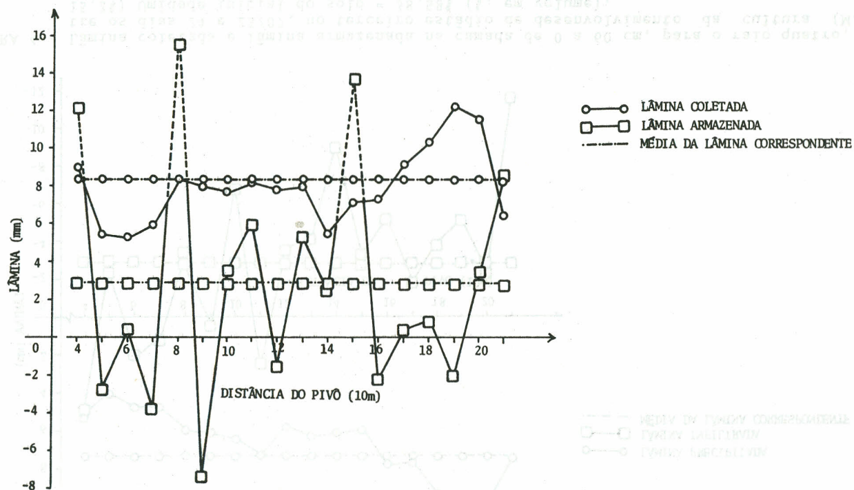
FIGURA 5 - Lâmina coletada e lâmina armazenada na camada de 0 a 60 cm, para o raio quatro, entre os dias 12 e 13/08, no terceiro estágio de desenvolvimento da cultura (M.S. = 18,2%). Umidade inicial do solo = 33,84% (% em volume).
