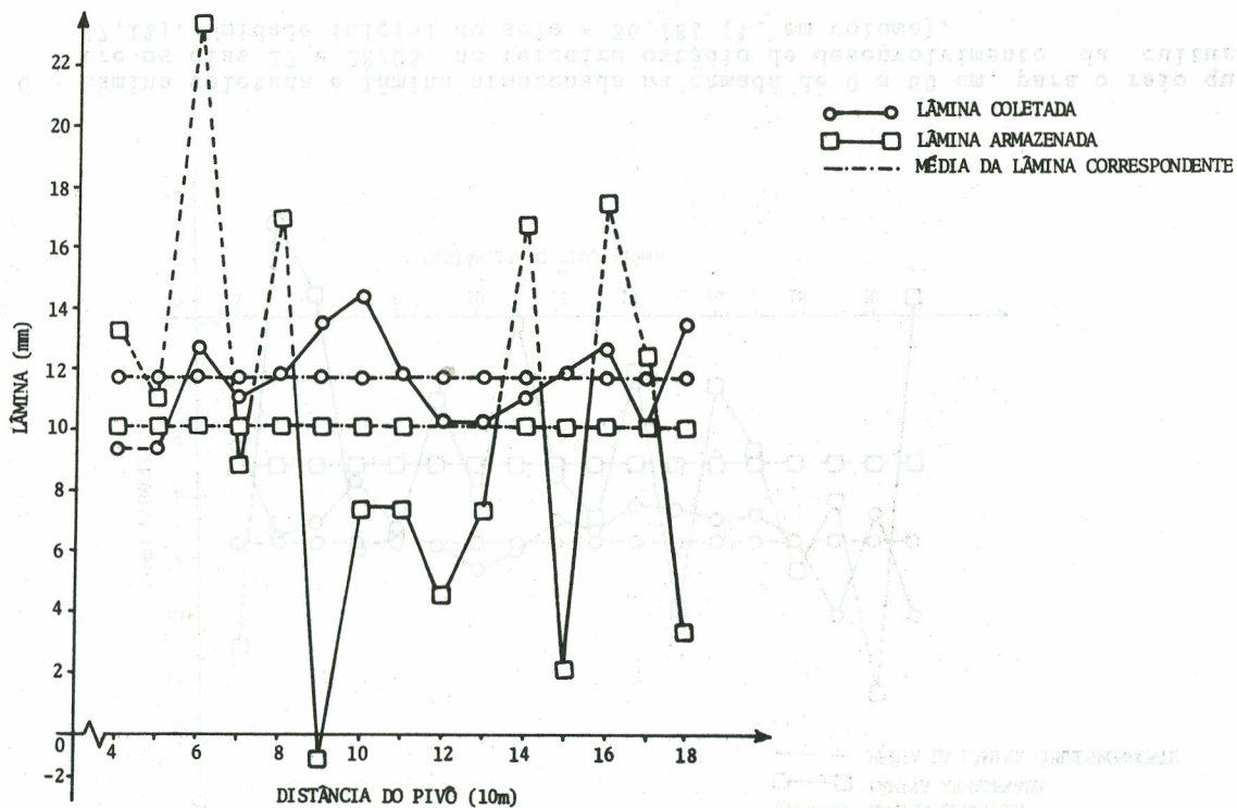
FIGURA 7 - Lâmina coletada e lâmina armazenada na camada de 0 a 60 cm, para o raio um, entre os dias 09 e 10/06, no primeiro estágio de desenvolvimento da cultura (M.S. = 0,0%). Umidade inicial do solo = 32,70% (% em volume).
