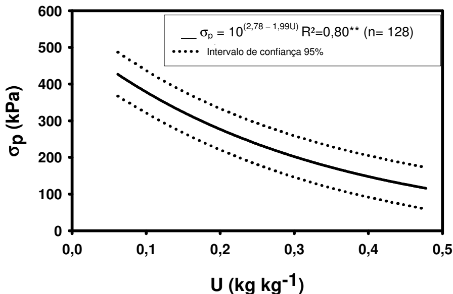
Figura 1. Modelos da capacidade de suporte de carga para o Latossolo Amarelo (Região Rio Doce) na profundidade de 10-13 cm. Fonte: (Dias Junior et al., 2005).
