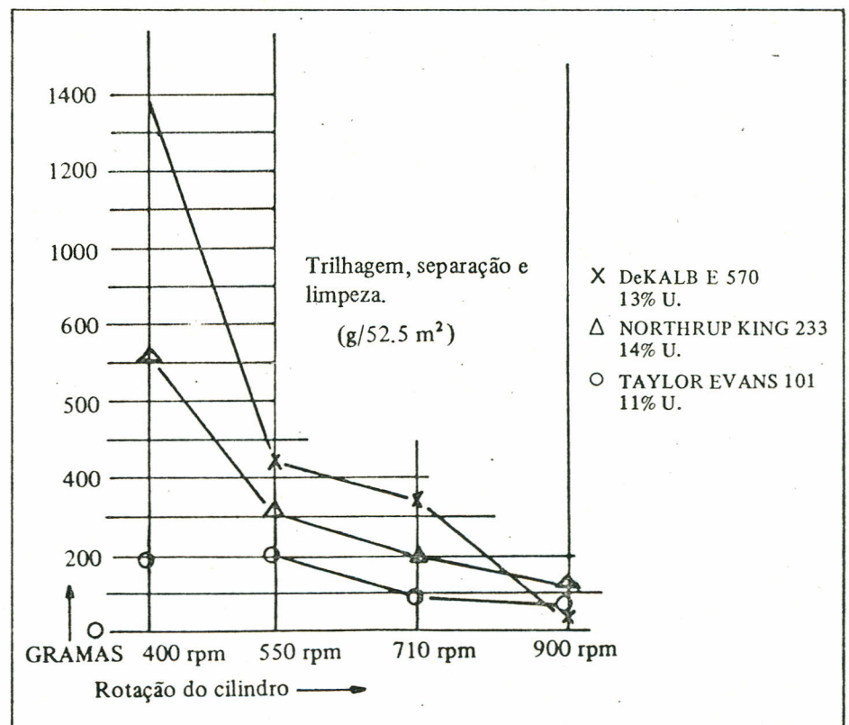
Fig. 3 - Perda em três variedades em relação à rotação do cilindro.
