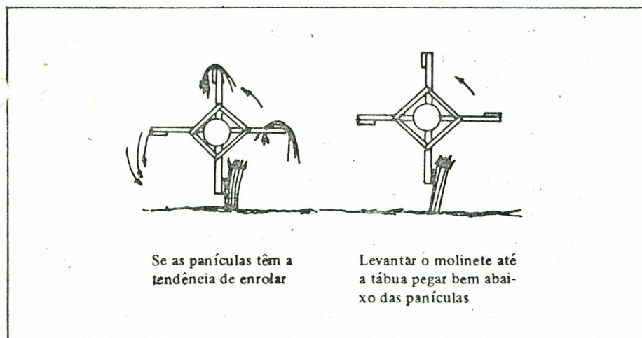
Fig. 5 – Ajuste da altura do molinete.
