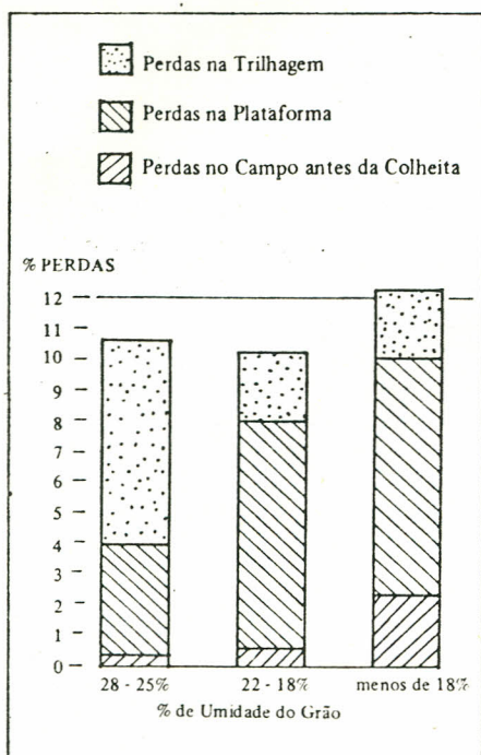
Fig. 4 – Limites máximos de perdas de grãos na colheita de sorgo.
