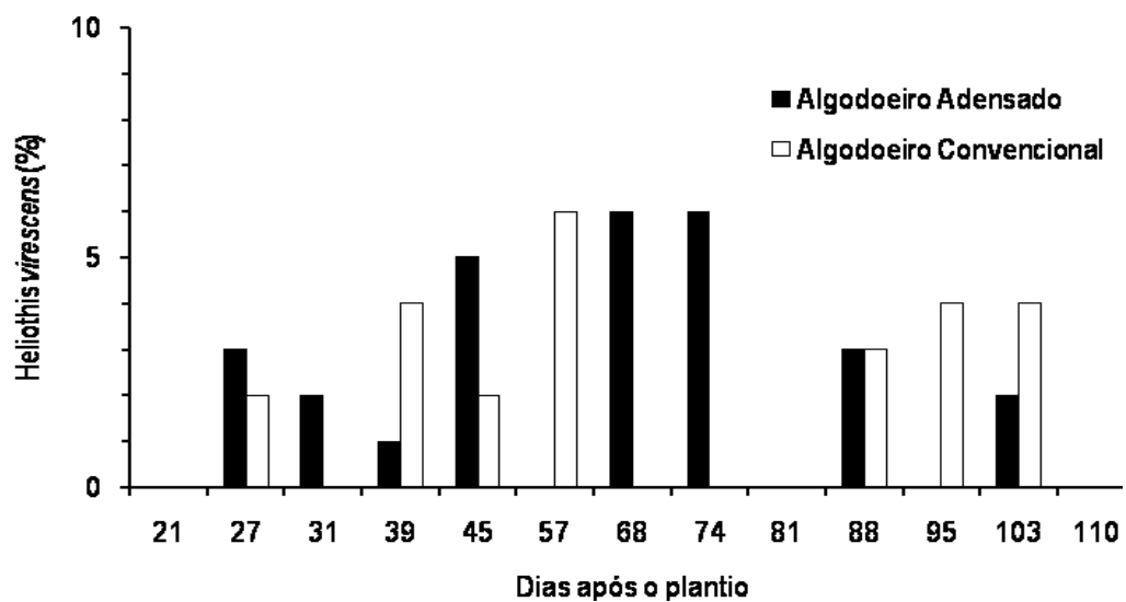
Figura 3. Incidência de Heliothis virescens nos sistemas de plantio adensado e convencional de algodoeiro (cultivar CD 408). Primavera do Leste (MT), 2009. Não significativo pelo teste de Fisher ( P=0,05 ).
