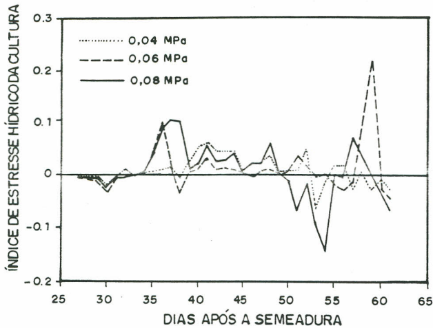
Figura 1 - Variação do Índice de Estresse Hídrico da Cultura do feijoeiro versus dias após a semeadura, para os tratamentos submetidos às tensões de 0,04; 0,06 e 0,08 MPa. Sete Lagoas, MG, 1993.
