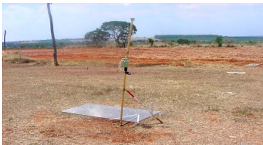
Figura 3.8. Placa de vidro com área de 0,75 m 2 e os sensores usados na medição da radiação solar interceptada pela palhada.
