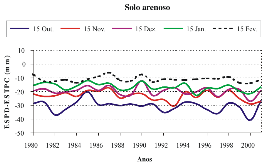
Figura 4.50. Diferença entre a evaporação da água de um solo textura média nos sistemas plantio direto (ESPD-mm) e convencional (ESPC-mm) para cinco datas de plantio em Passo Fundo-RS.
