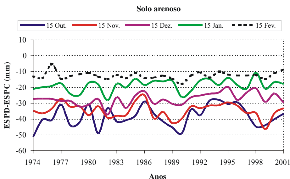
Figura 4.43. Diferença entre a evaporação da água do solo textura média nos sistemas plântio direto (ESPD-mm) e convencional (ESPC-mm) para cinco datas de plântio em Planaltina-DF.
