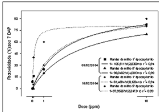
Figura 1 – Porcentagem de fitotoxicidade visual nas plantas de milho BRS 3003 aos 7 dias após plantio (DAP), detectadas a partir das diferentes doses de diclosulam incorporadas ao solo, nos experimentos 1 e 2. Embrapa Milho e Sorgo, Sete Lagoas, MG, 2004.
