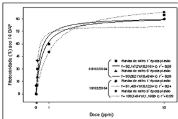
Figura 2 - Porcentagem de fitotoxicidade visual nas plantas de milho BRS 3003 aos 14 dias após plantio (DAP), detectadas a partir das diferentes doses de diclosulam incorporadas ao solo, nos experimentos 1 e 2. Embrapa Milho e Sorgo, Sete Lagoas, MG, 2004.
