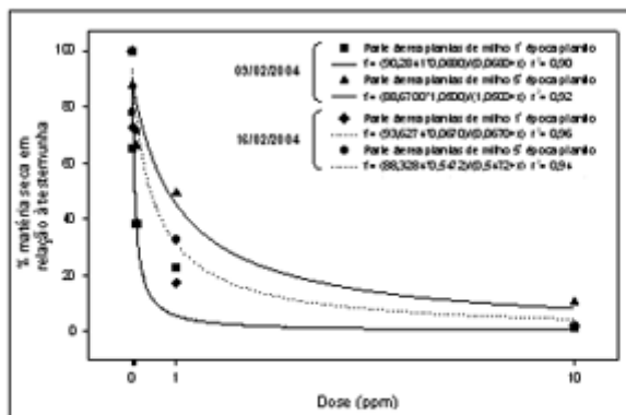
Figura 3 – Porcentagem de matéria seca de milho plantado nas diferentes doses do herbicida diclosulam incorporadas ao solo, em relação à testemunha, nos experimentos 1 e 2. Embrapa Milho e Sorgo, Sete Lagoas, MG, 2004.
