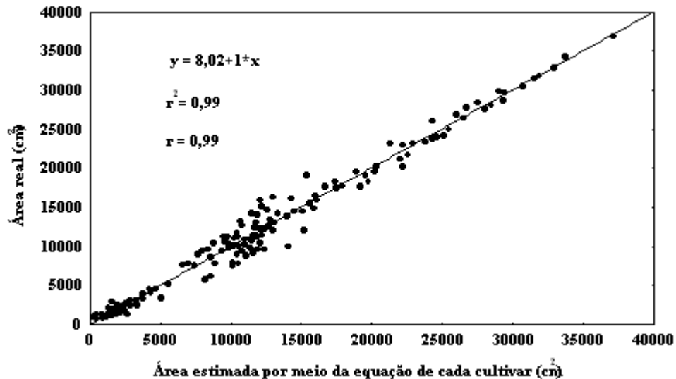
Figura 3. Relação entre os valores da área estimada pela equação de cada cultivar e a área real nas duas épocas de coleta. Embrapa Milho e Sorgo. Sete Lagoas, MG. 1993
