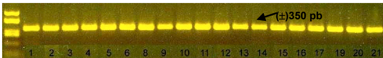
Figura 1. Gel de agarose com fragmentos do fator de lacrimejação presente em plantas da cultivar de cebola BRS Alfa São Francisco. A primeira coluna do lado esquerdo é o padrão de 50 pb da Amresco DNA MicroMarker. Petrolina, PE, 2005.
