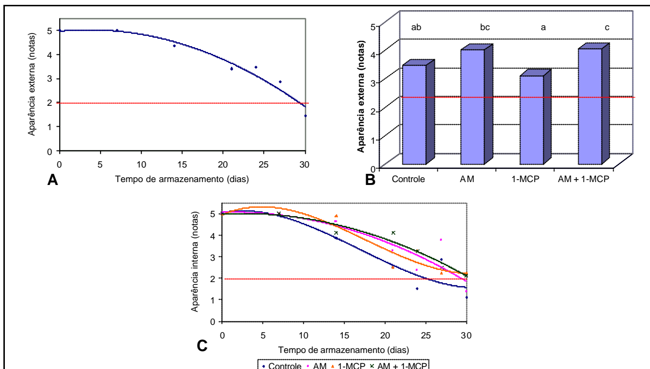
Figura 2. Aparência de melão Galia 'Solar King' submetido a atmosfera modificada (AM) e à aplicação de 1-MCP, durante 21 dias de armazenamento refrigerado ( 7,6\pm 1,1^{\circ}\text{C} e 87,6\pm 6,3\% UR) seguido de até 9 dias em temperatura ambiente ( 24,2\pm 0,7^{\circ}\text{C} e 88,1\pm 5,4\% UR). A linha vermelha paralela ao eixo x indica o limite de aceitação do fruto pelo consumidor.
