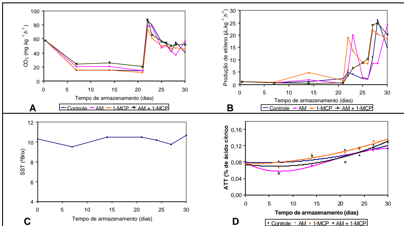
Figura 1. Atividade respiratória (A), produção de etileno (B), teor de sólidos solúveis totais – SST – (C) e acidez total titulável – ATT – (D) de melão Galia ‘Solar King’ submetido a atmosfera modificada (AM) e à aplicação de 1-MCP, durante 21 dias de armazenamento refrigerado (7,6±1,1°C e 87,6±6,3% UR) seguido de até 9 dias em temperatura ambiente (24,2±0,7°C e 88,1±5,4% UR).
