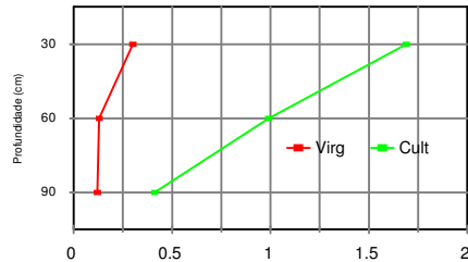
Fig. 2 - Variação dos valores de CE dS/m nos solos virgens e cultivados
