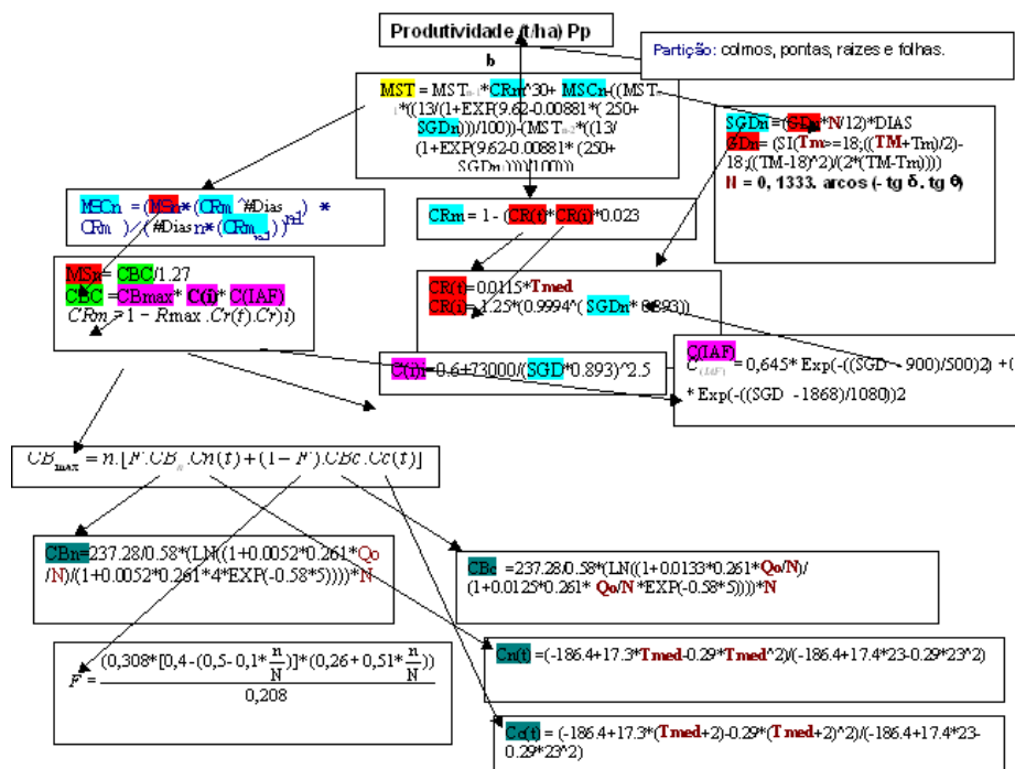
Figura 1. Fluxograma do modelo BRCANE proposto para estimar a produtividade potencial da cana-de-açúcar em função do clima.
