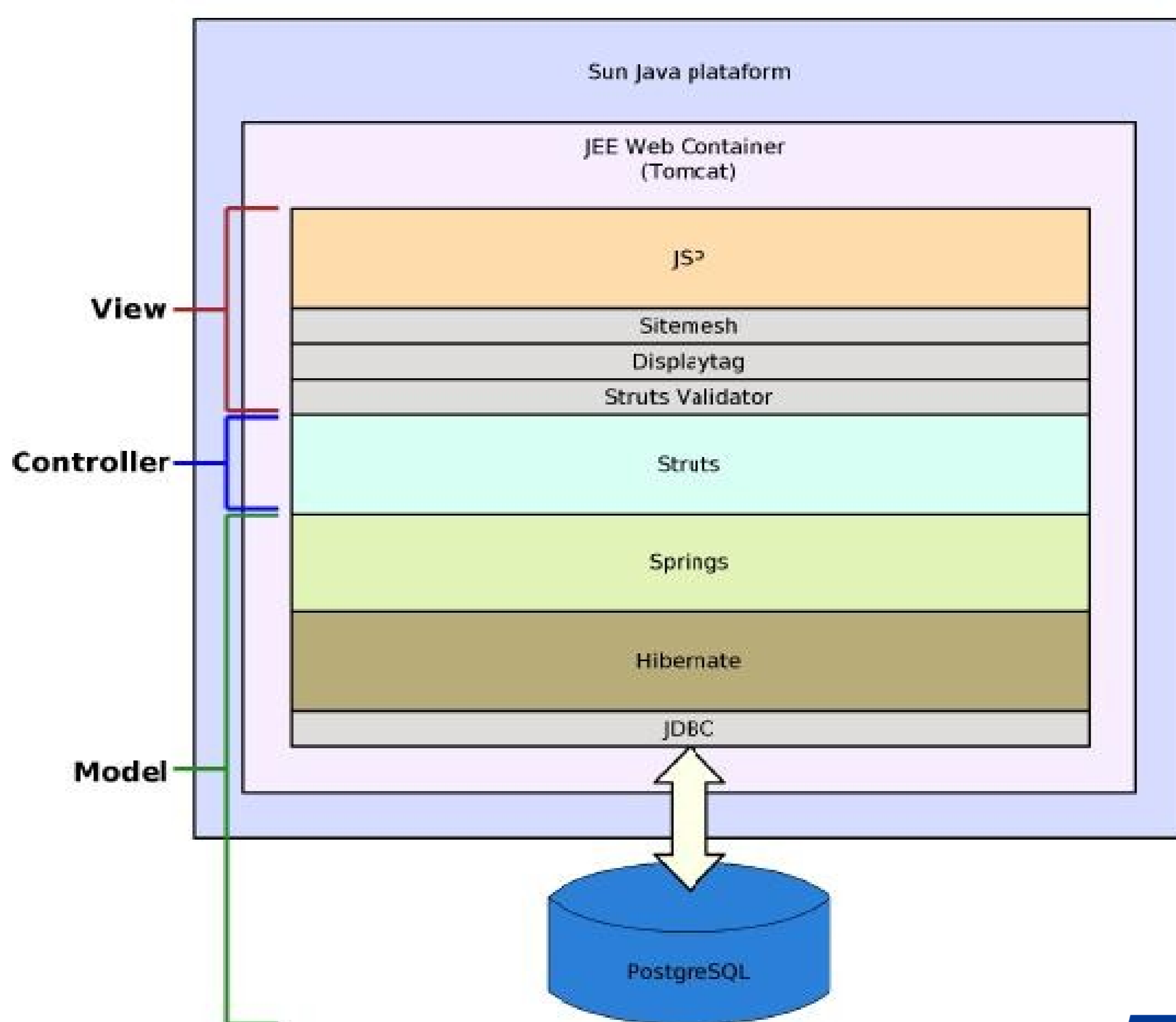
Figura 1. Plataforma de software utilizada no sistema
