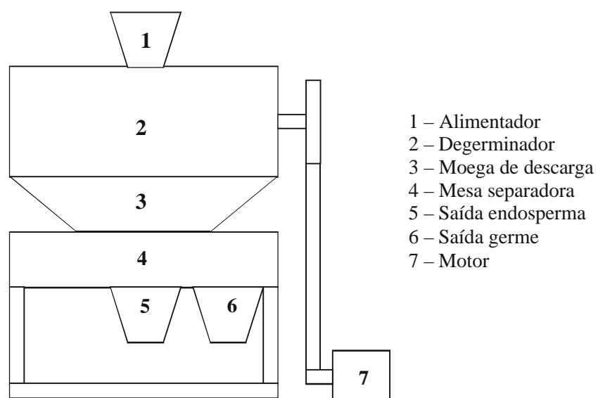
FIGURA 1 – Degerminador de facas.
