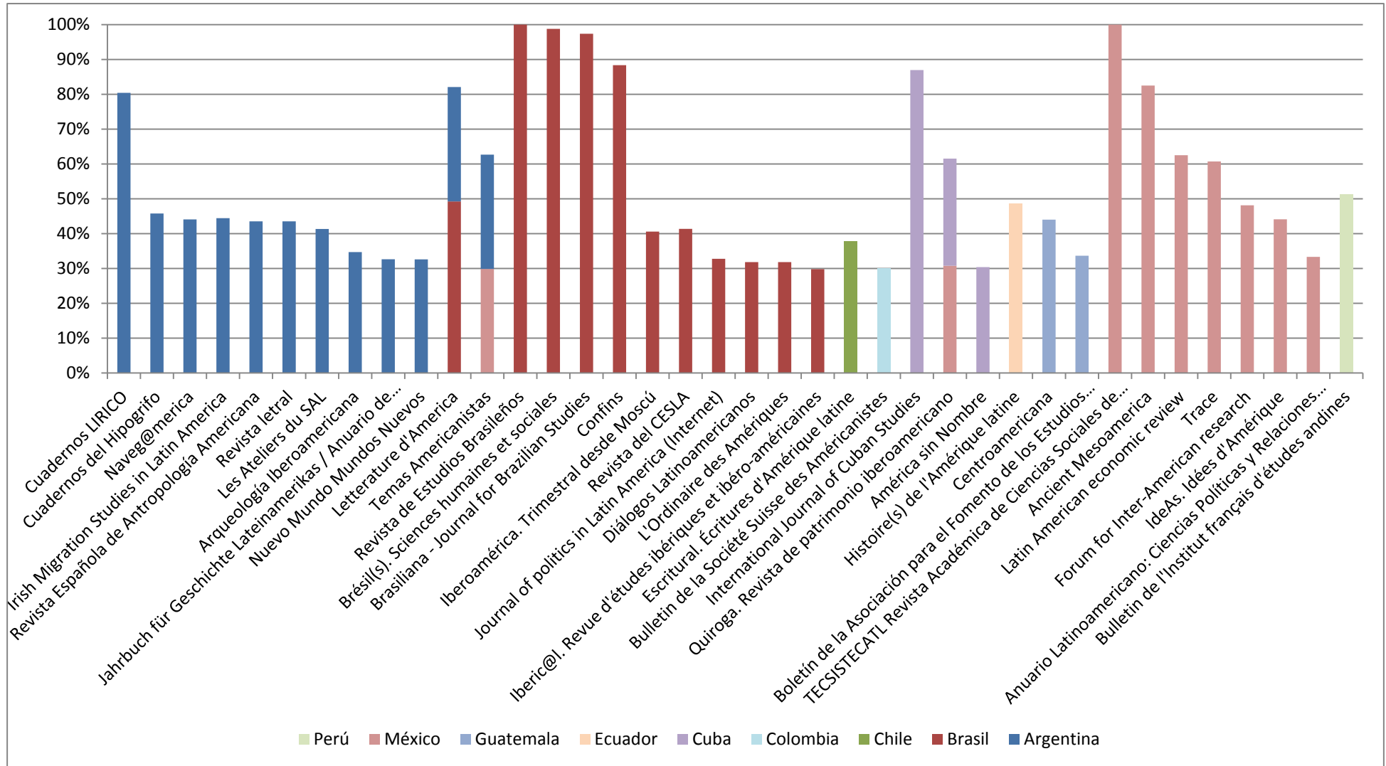
Figura 4: Palabras geográficas de 30% o más por país y revista
