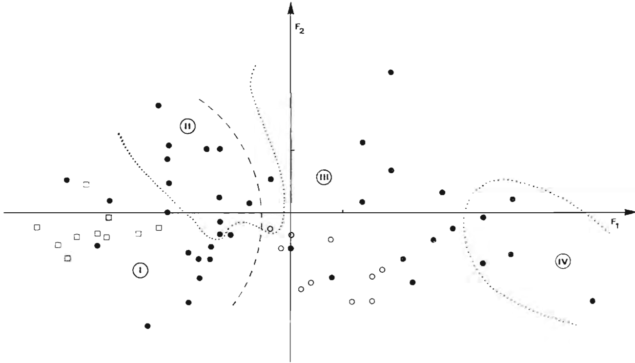
Fig. 5. Analyse en Composantes Principales normés après élimination des C. bolivari — 9 variables mandibulaires. Représentation du plan factoriel F_1F_2 . F_1 : taille décroissante, F_2 : variations de P2 et BM (symboles de la fig. 4). Analyse taxinomique: la 1ère partition (en tirets) sépare le groupe I-II (dont C. russula ) de III-IV (dont C. whitakeri ), la 3ème partition (en pointillés) isole deux classes dans ces deux ensembles dont la classe IV regroupant des mandibulees de très petite taille.
