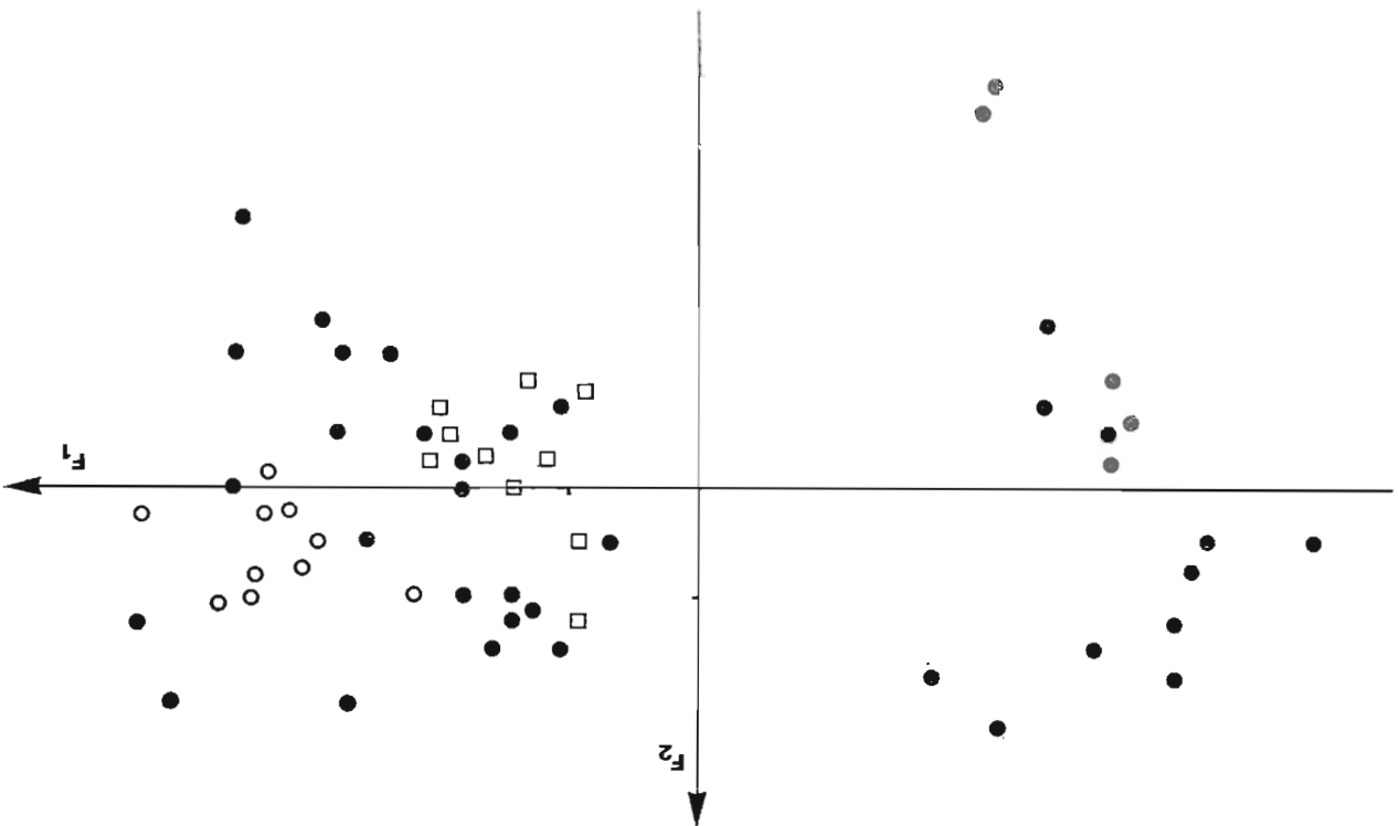
Fig. 2. Analyse en Composantes Principales normée — 12 variables crâniennes. Représentation du plan factoriel F_1F_2 . F_1 est un facteur de taille décroissante, F_2 est lié à la hauteur de la P^4 et de son paracône; ronds noirs: spécimens de Massa; ronds blancs: C. whitakeri (Marrakech); carrés blancs: C. russula (Marrakech).
