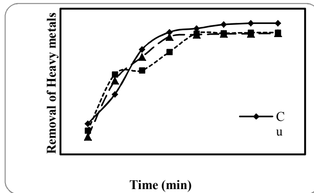
شکل شماره ۱. راندمان حذف فلزات سنگین در زمان واکنش مختلف، pH شیرابه (pH=7.4)، دانسیته جریان 110 \text{ mA/cm}^2 هدایت الکتریکی 60 \text{ ms/cm}
