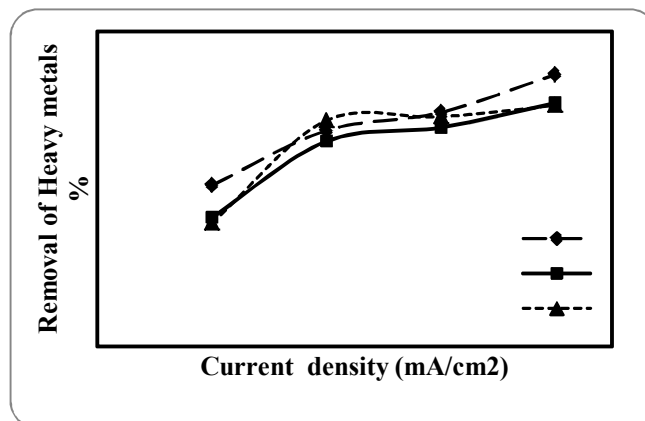
شکل شماره ۲. راندمان حذف فلزات سنگین در دانسیته جریان مختلف، زمان ۲۵ دقیقه pH شیرابه (pH=7.4)، هدایت الکتریکی 60 \text{ ms/cm}
