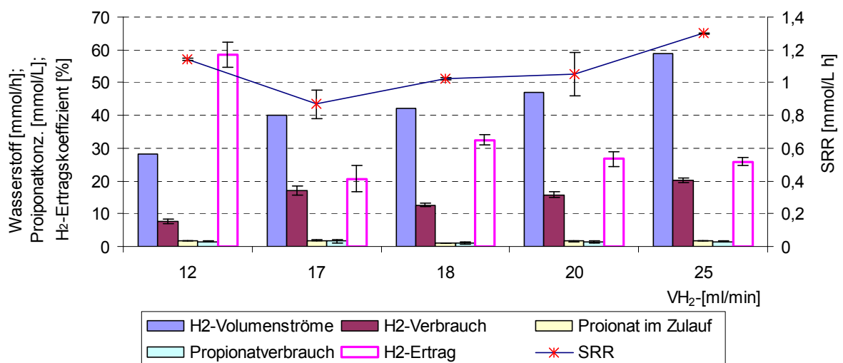
Abb. 4.2-12: Beziehungen zwischen H 2 -Volumenströmen und Wasserstoffertagskoeffizienten bei der VWZ von 0,33 Tagen
