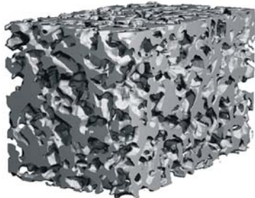
Das Bild zeigt einen Keramikschaum auf Basis eines präkeramischen Polymers
