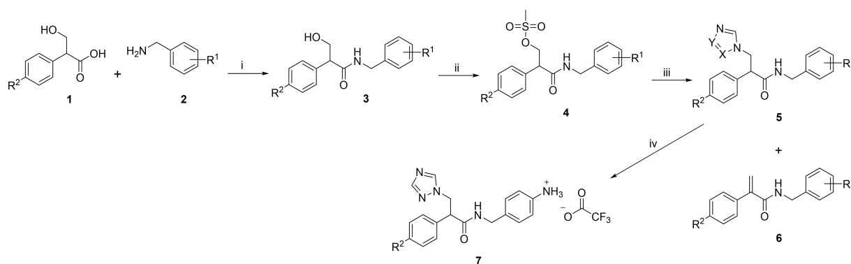
Scheme 1. i) B(OCH_3)_3 , CPME, 4 Å molecular sieves, 100 °C, o/n; ii) MsCl , Et_3N , CH_2Cl_2 , o/n; iii) a) K_2CO_3 , imidazole/triazole/tetrazole, CH_3CN , 45 °C, 1 h; b) 4, 70 °C, 1–24 h; iv) 5I , TFA, CH_2Cl_2 .
