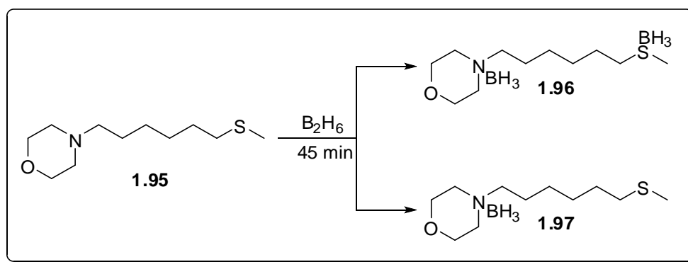
Scheme 1.34
