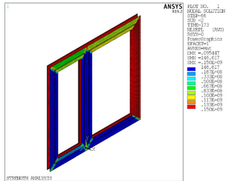
(d) Plastic equivalent stress
