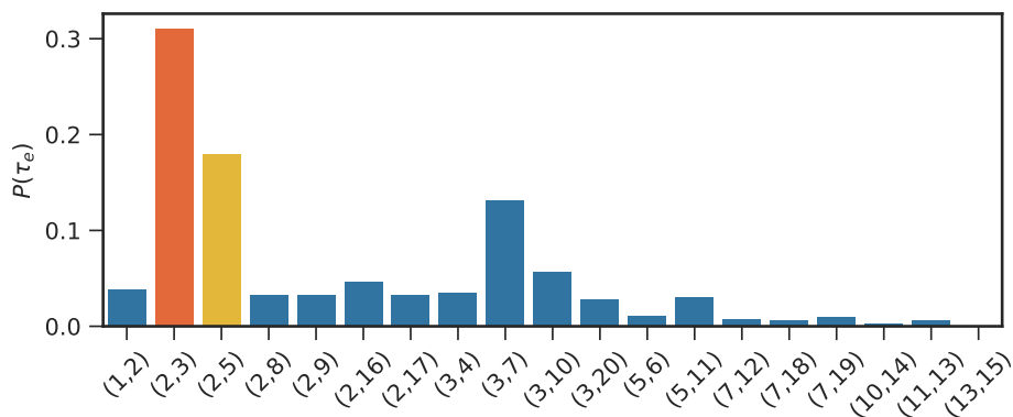
FIGURE 1.5 – (haut) Réseau artificiel de N = 20 noeuds, généré par le processus d’attachement préférentiel avec un exposant \gamma = 1 . Les chiffres apparaissant sur les noeuds indiquent leur ordre d’arrivée. (bas) Estimation empirique de P(\tau_e = 1) , i.e., la probabilité que le lien e soit apparu le premier.
