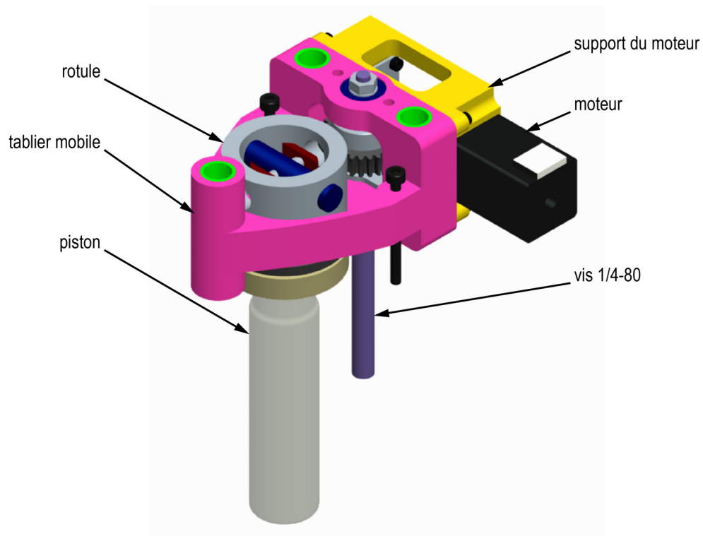
Figure 3.12 : Modélisation du sous-assemblage du chariot.
