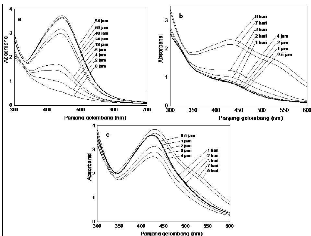
Gambar 2 Spektra serapan UV-Vis AgNPs selama waktu inkubasi dengan suhu (a) 30, (b) 60, dan (c) 90 °C
