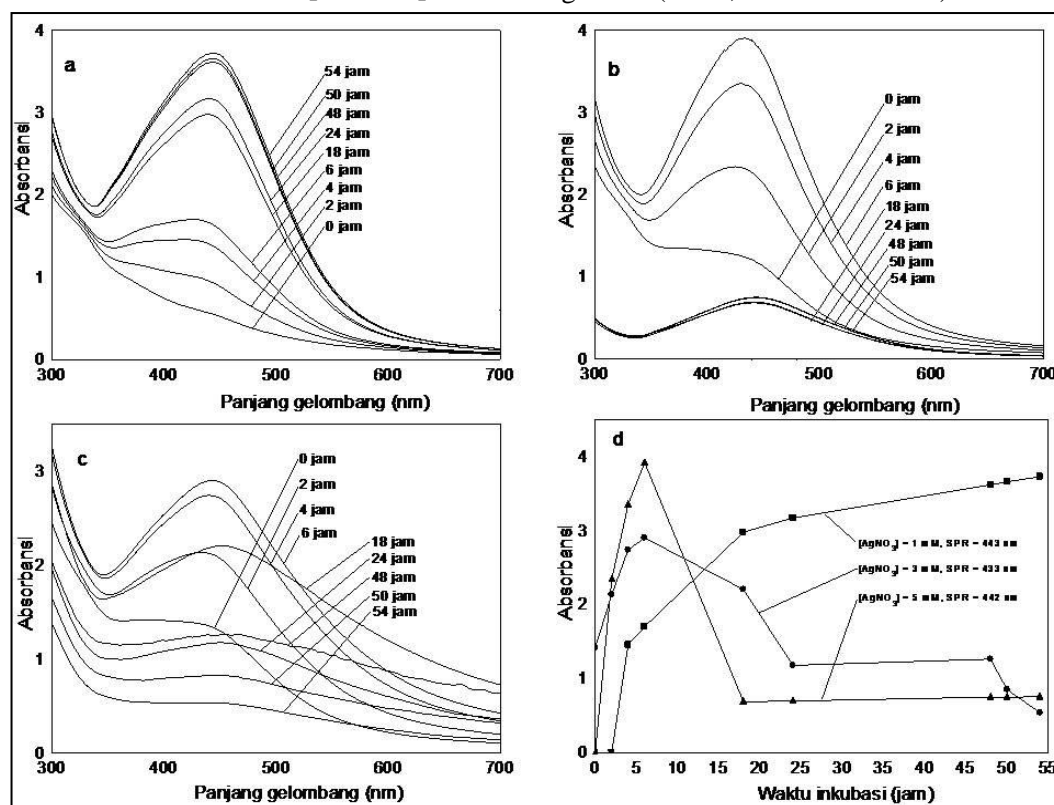
Gambar 1 Spektra serapan UV-Vis AgNPs selama waktu reaksi dengan mereduksi masing-masing (a) 1, (b) 3, dan (c) 5 mM larutan AgNO 3 menggunakan ekstrak kulit buah manggis 0.015 g/mL. (d) perubahan intensitas serapan SPR selama waktu reaksi.
