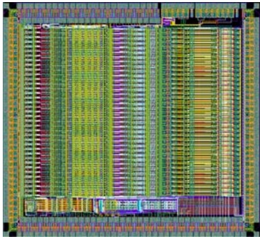
Fig. 2 – SKIROC layout
