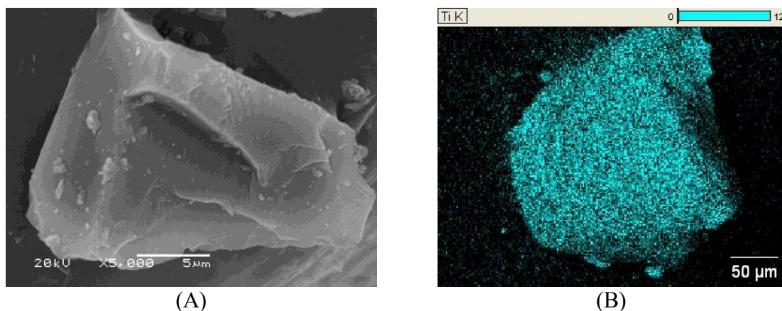
Figura 1. Micrografía de ladrillo reciclado de suelo cemento: (A) con detector de imágenes de electrones secundarios (B) Imagen obtenida con EDS para Ti.
