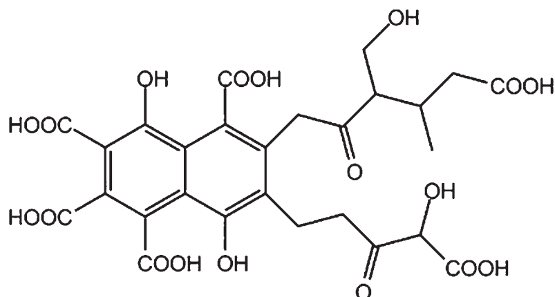
Рис. Структурная формула фульвово́й кислоты (479-66-3).
