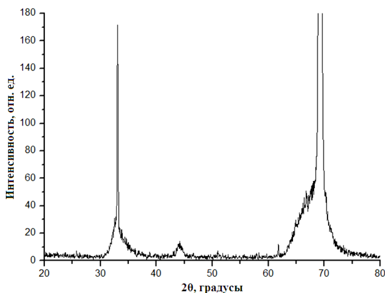
Рис. 3. Дифрактограмма пятислойной пленки титаната стронция, подвергнутой термообработке при температуре 750 °С в течение 30 мин
