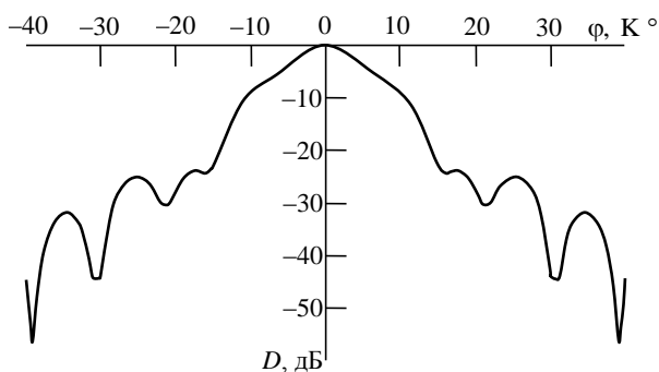
Рис. 5. Диаграмма направленности тороидально-бифокальной линзовой антенны с одной преломляющей поверхностью в горизонтальной плоскости (результаты электромагнитного моделирования)
