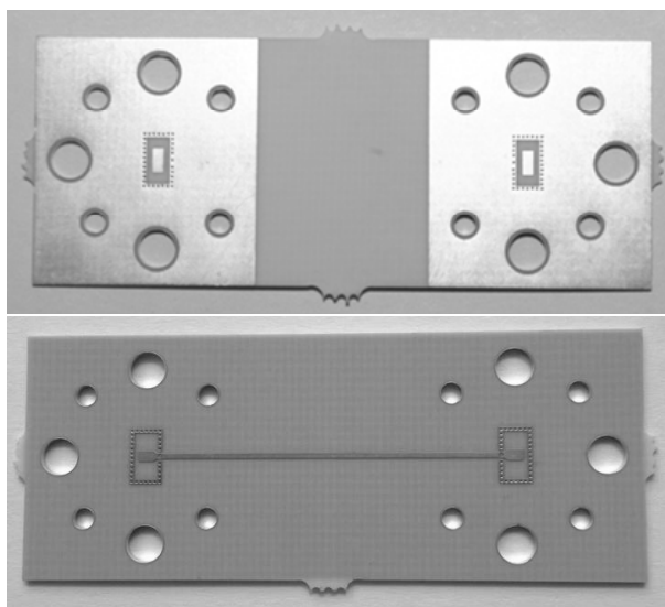
Рис. 8. Макет печатной платы с двусторонним переходом "волноводно-микроразветвляющая линия-волноводно"
