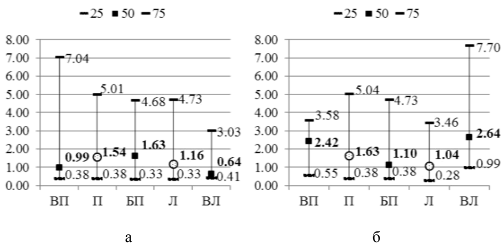
Рис. 11. Аналіз (Med, Q 1 , Q 3 ) даних виміру ЧРС (л) у чоловіків (а) та жінок (б) з урахуванням моторної асиметрії: ВП – виражено праворукі, П – праворукі, БП – без переважання (амбідекстри), Л – ліворукі, ВЛ – виражено ліворукі.
