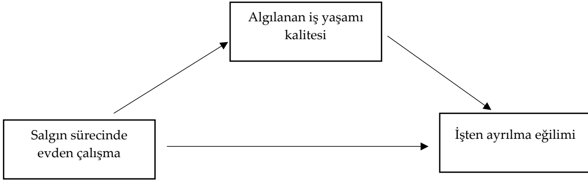
Şekil 1. Araştırmanın modeli
