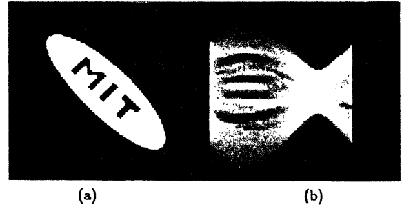
Fig. 5. MIT ellipse and noise-free sinogram.
